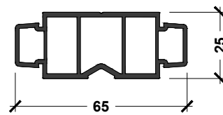
APX.ANC.061 THERMAL CORE 1
