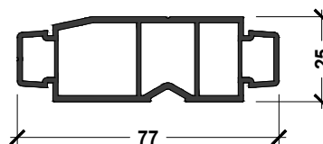
APX.ANC.062 THERMAL CORE 2
