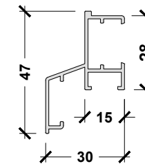
APX.ANC.101 VENT HOOD
