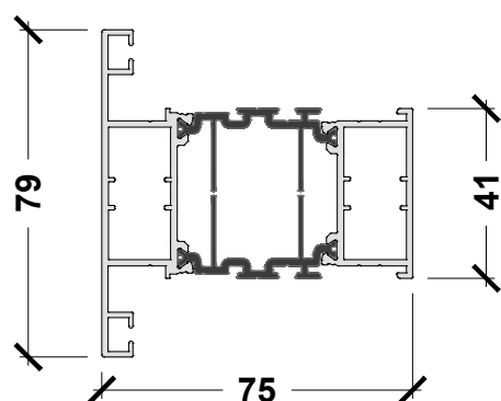
APX.DRT.079 79MM DOUBLE REBATE T
