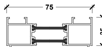
APX.ANC.200 25MM ADD-ON (STANDARD)
