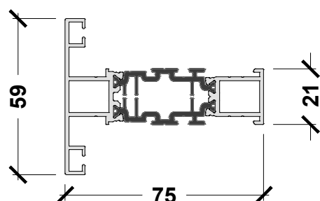
APX.DRT.059 59MM DOUBLE REBATE T
