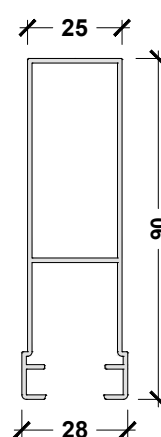
APX.ANC.091 HD BOLSTER
